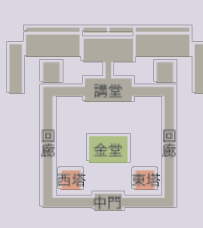
◎薬師寺式伽藍配置図
